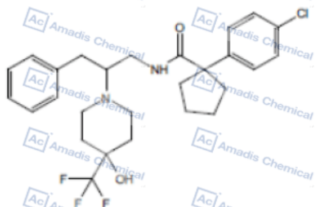
GDM-312-B 400MHz 1H-NMR DMSO-d 6
