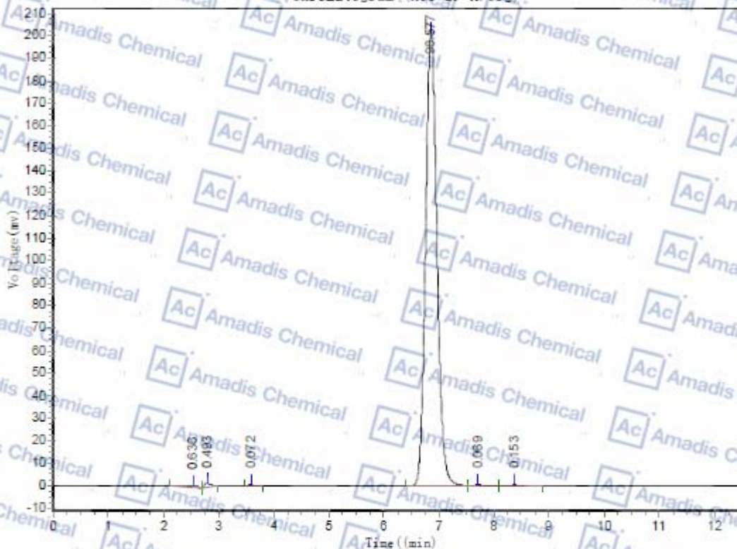
Chromatogram (VATS-EP-A.ora)
